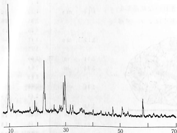
図9 輝沸石の粉末X線回折曲線
