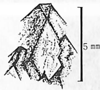
図12 ギョガン石
