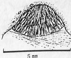
図3 方沸石
