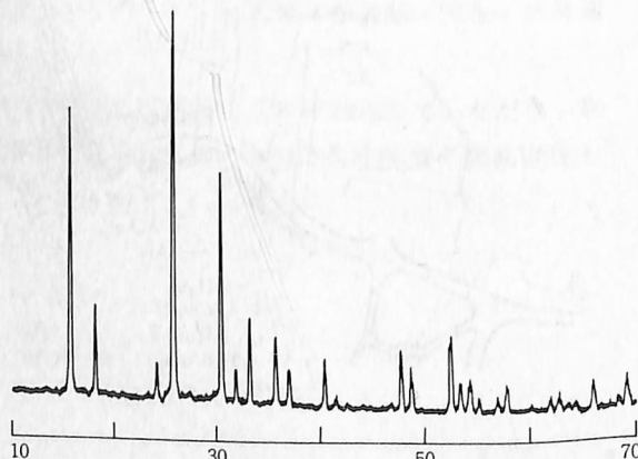
図4 方沸石の粉末X線回折曲線
