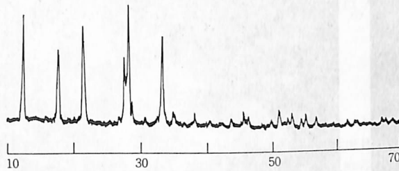
図11 灰十字沸石の粉末X線回折曲線
